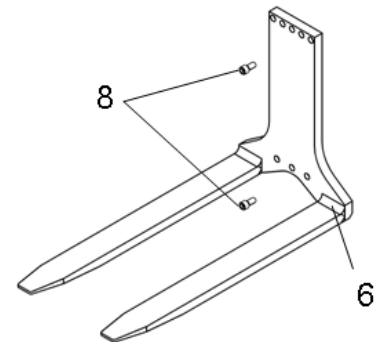
Modell T491W/180
