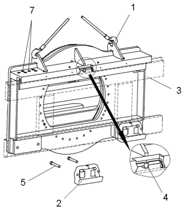
mit Seitenschub
