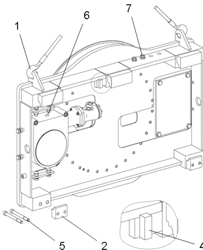
ohne Seitenschub
